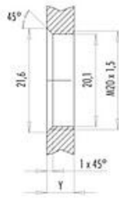
Mit Durchgangsbohrung
